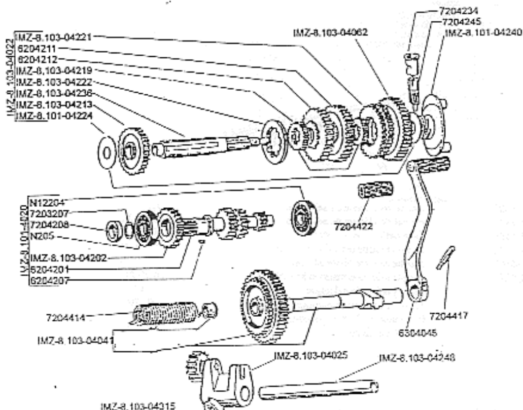
Fig10.Pignonnerie boite de vitesse
