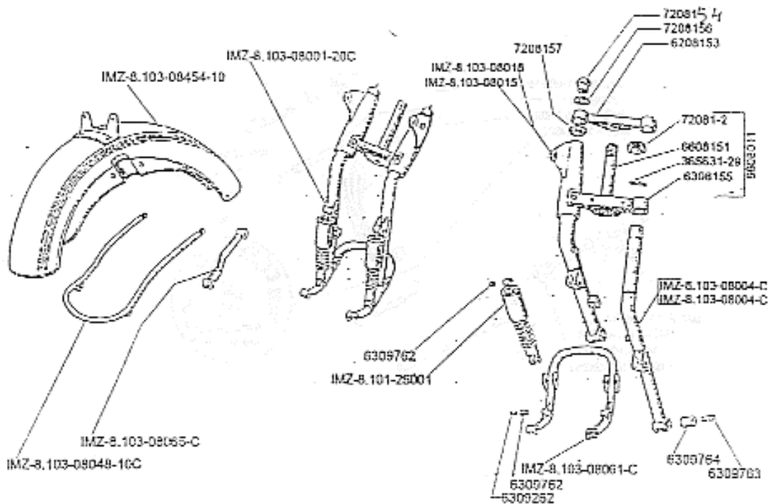
Fig19.Fourche a balancier
