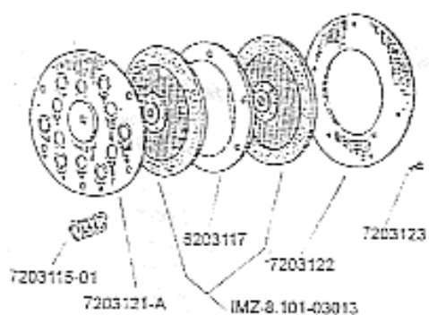
Fig7.Embrayage
