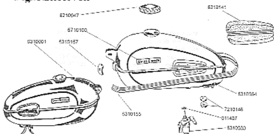
Fig25. Reservoir
