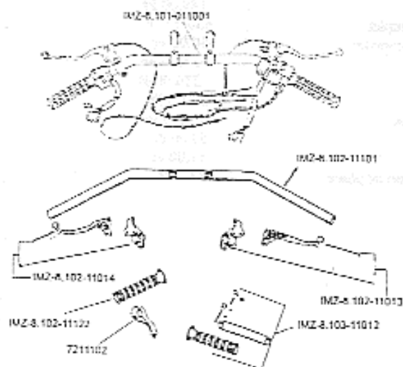
Fig22.Guidon
