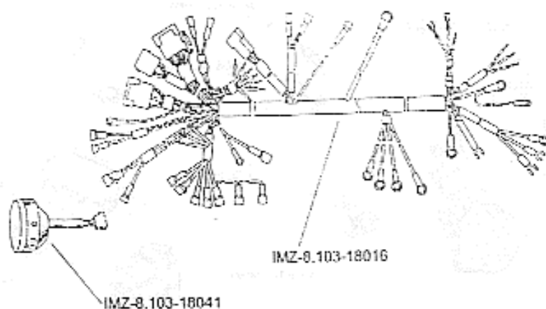
Fig27.Faisceau electrique
