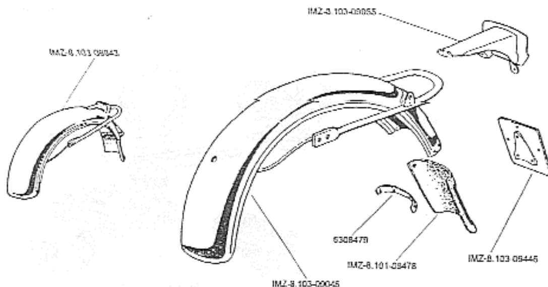
Fig24. Garde boue arriere
