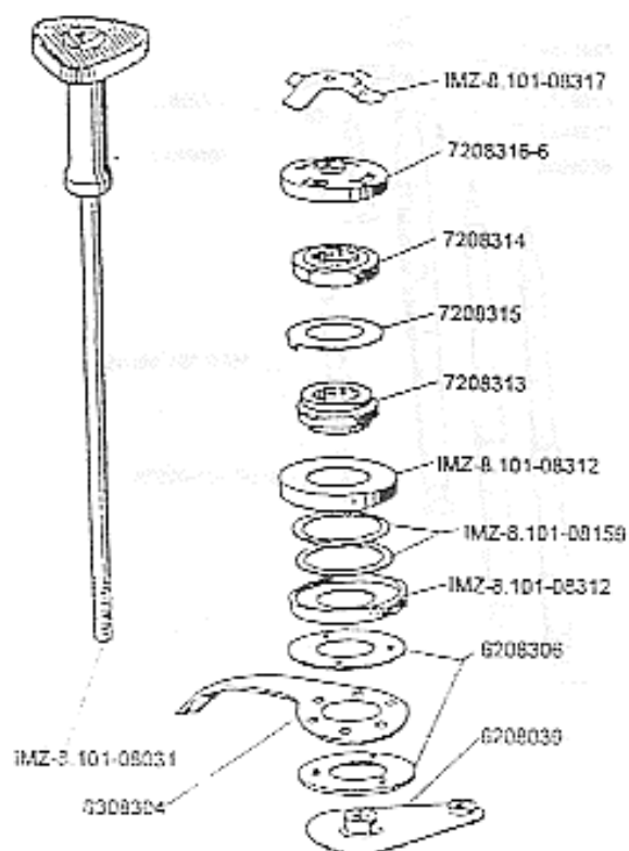
Fig22.Guidon
