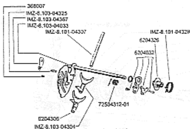
Fig11.Mecanisme de selection
