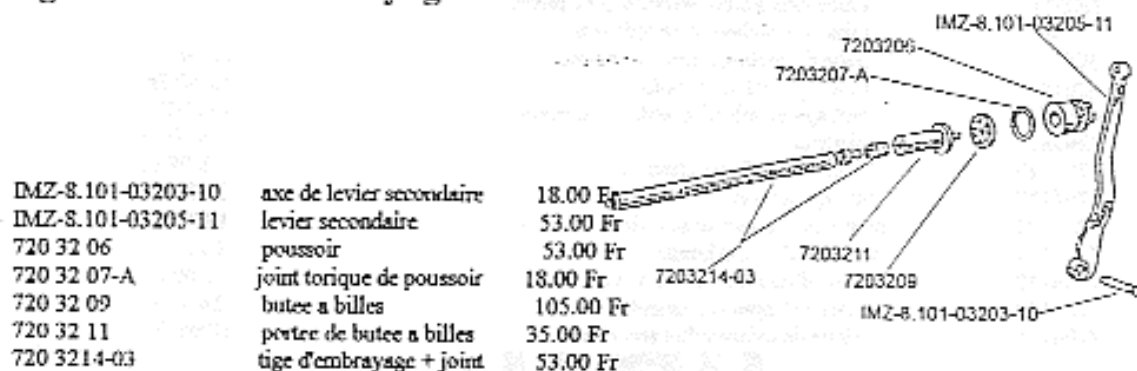
Fig8.Commande embrayage
